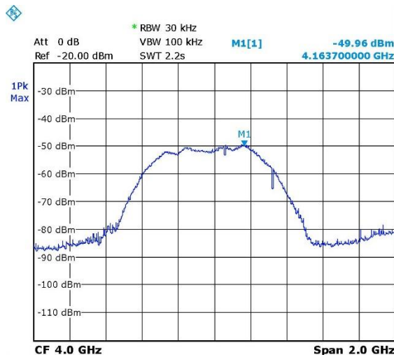
图 1.3.3 UWB Mini 4 发射功率测试
