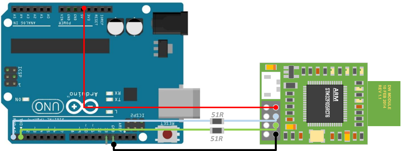
图 6.7.3 UWB Mini 4 模块与单片机(Arduino)相连
