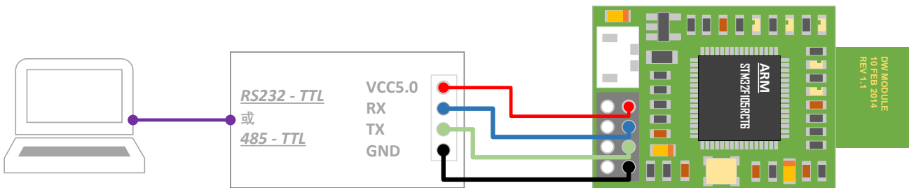
图 5.2 UWB Mini 4 模块与 TTL 转 RS232 模块或 TTL 转 485 模块相连
