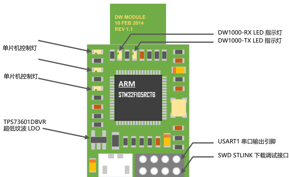
图 1.3.1.1 UWB Mini4 正面图
