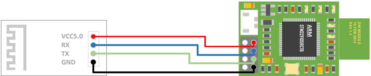
图 6.7.2 UWB Mini 4 模块与蓝牙模块相连
