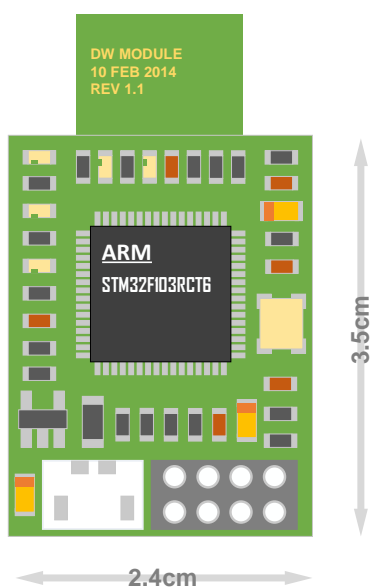
图 1.3.1.1 UWB Mini4 正面图
