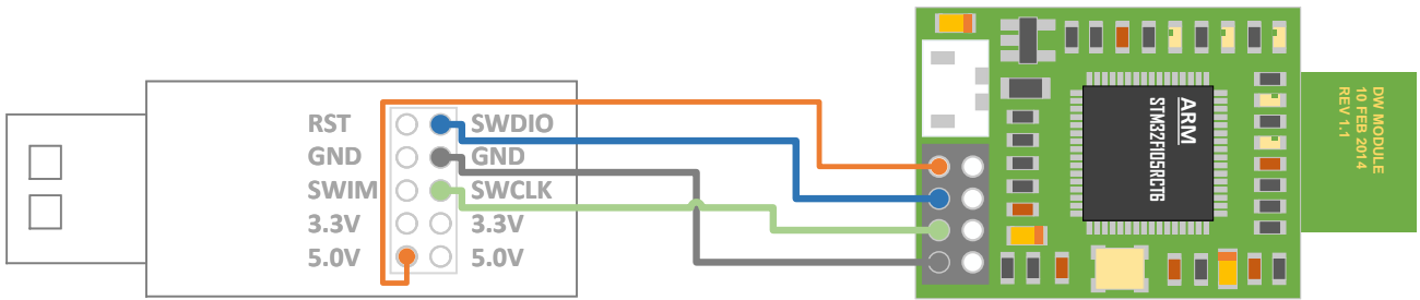
图 5.1 STLINK V2 下载器与 Mini4 硬件接线方法
